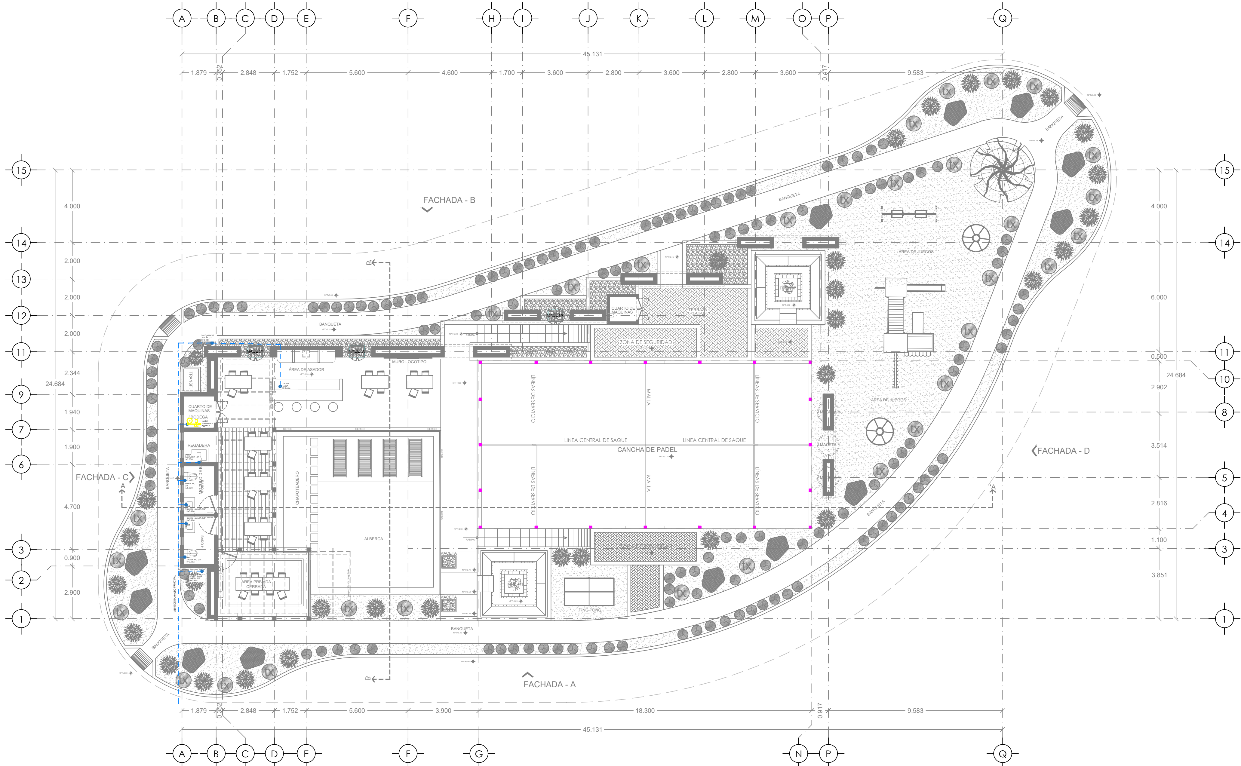
PLANTA DE INSTALACIÓN HIDRÁULICA ESC 1:125
